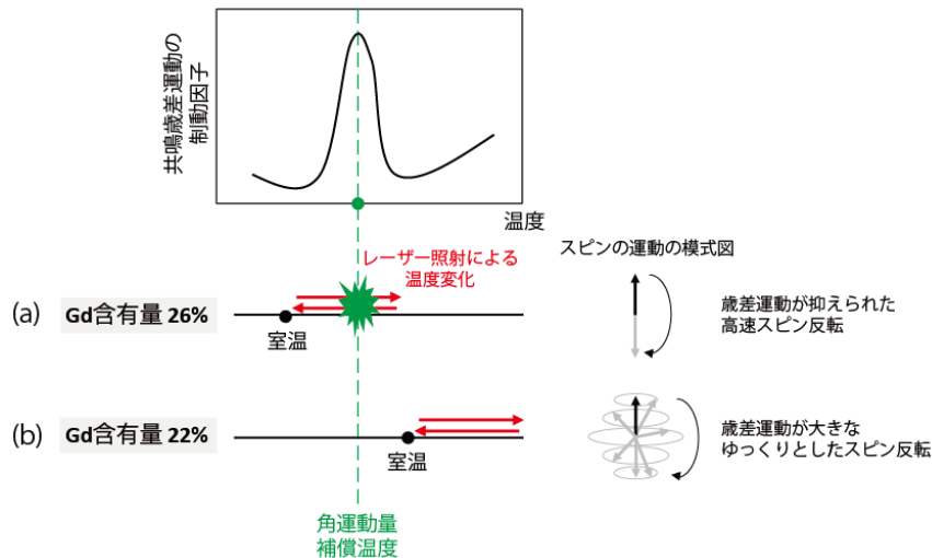
図 3. パルスレーザー光が照射された時に予想される Gd-Fe-Co 薄膜のスピンの運動の概念図。(a)Gd 含有量 26%の試料では角運動量補償温度が室温より高く、歳差運動の抑制因子が大きくなる温度領域を通過するため、高速なスピン反転が実現されます。(b)Gd 含有量が 22%の試料では角運動量補償温度が室温より低く、レーザー励起による歳差運動の抑制が小さいため、スピン反転時間は間延びします。Gd-Fe-Co 薄膜系におけるこれまでの研究では、(a)の条件での高速スピン反転が注目されていましたが、今回の研究では、(b)の条件において巨大なスピン波を新規に見出しました。
