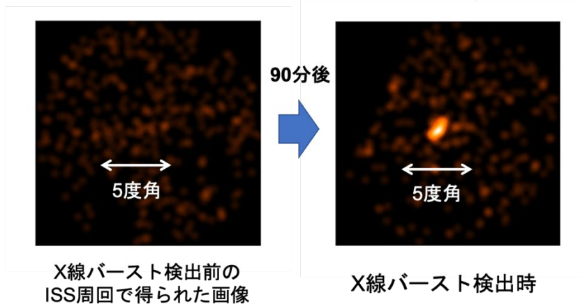
図 2 MAXI による M15 の X 線画像(X 線バースト検出前と検出時)
