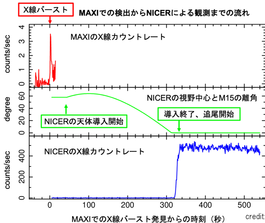
図 3 X 線バーストの発見から観測までの流れ
