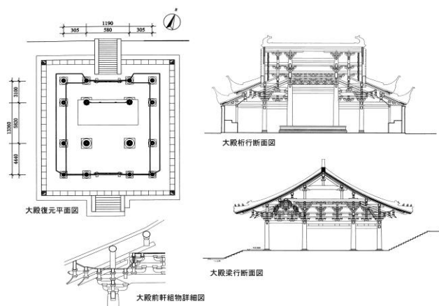
図-1 保国寺復元図 (保国寺 4) 文物出版社 2003 に加筆)
