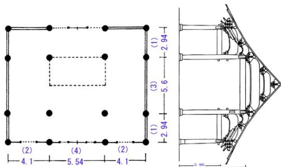
図-2 揚湾廟正殿平面・断面図 (参考文献1に加筆)
