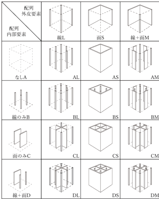
図2 架構材の構成と配列
