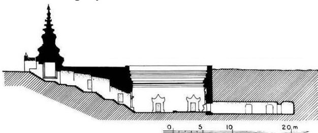
図3 Taung-Kyanzittha-umin の断面図 [2]
